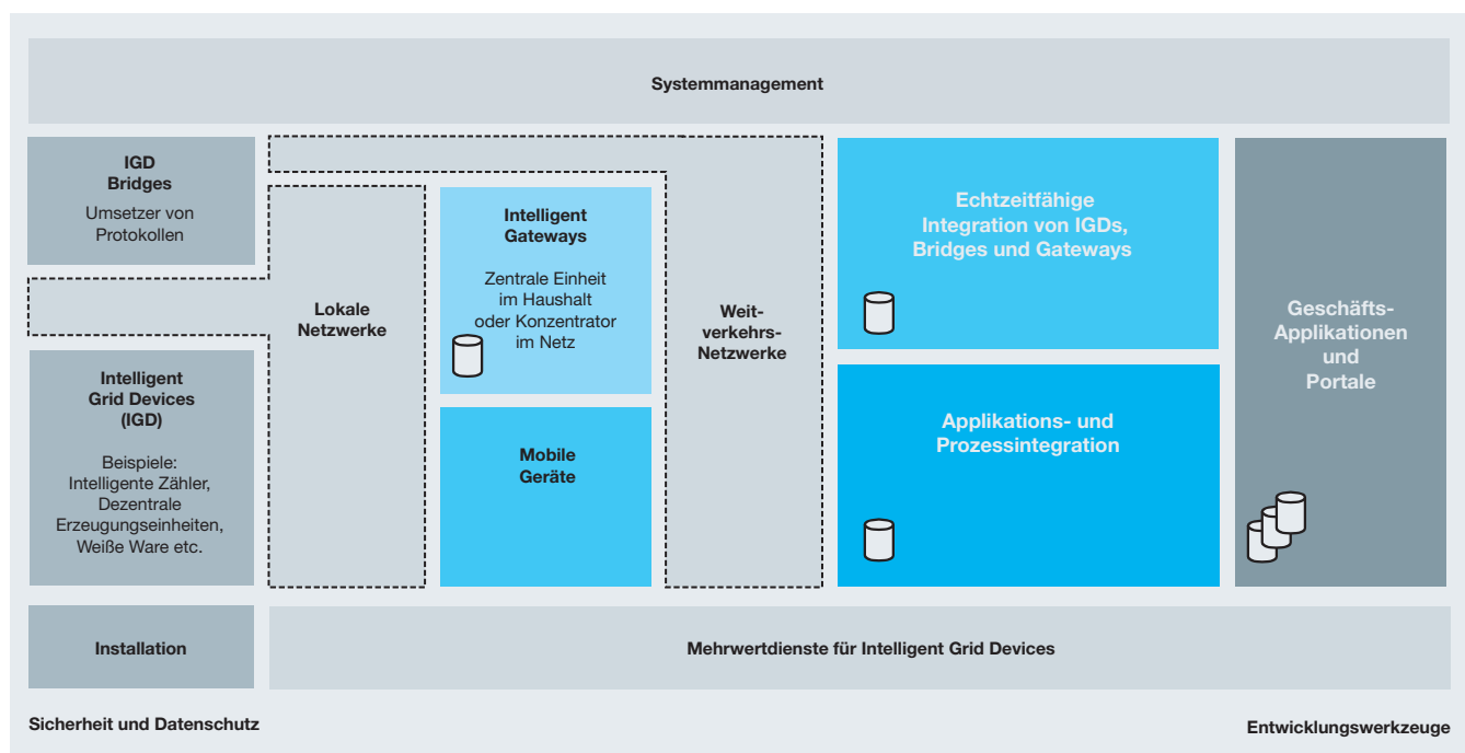
Abbildung 10: Anforderungsdomänen Internet der Energie
